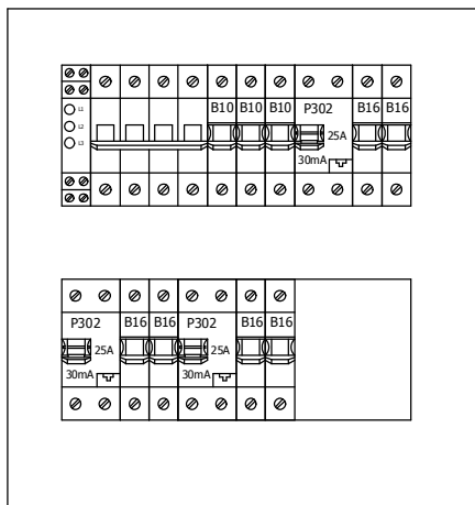
Rozdzielnica RP 2x12mod
